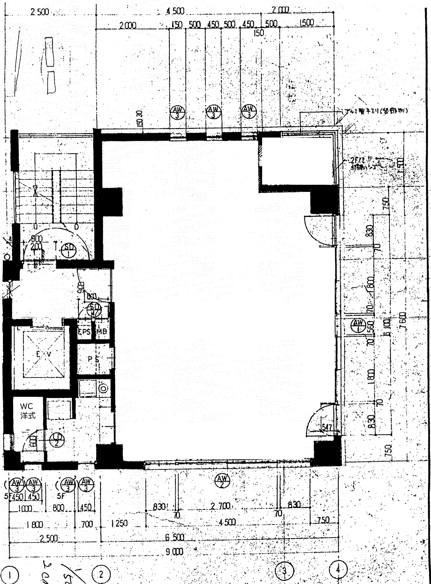
2~5F 平面詳細図
